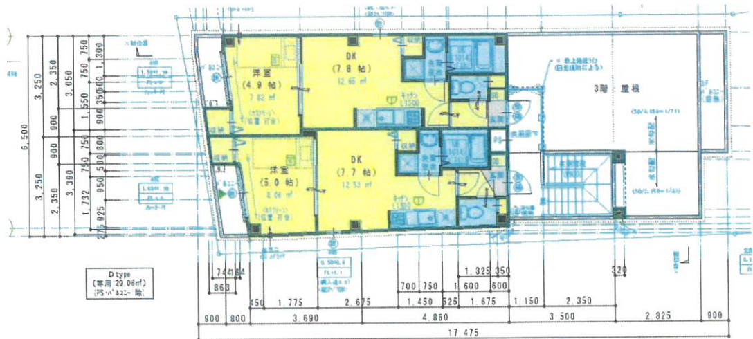
【4F 平面图】
