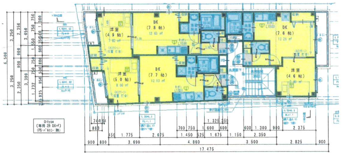
【2F 平面图】
