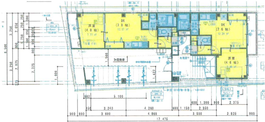
【1階 平面图】
